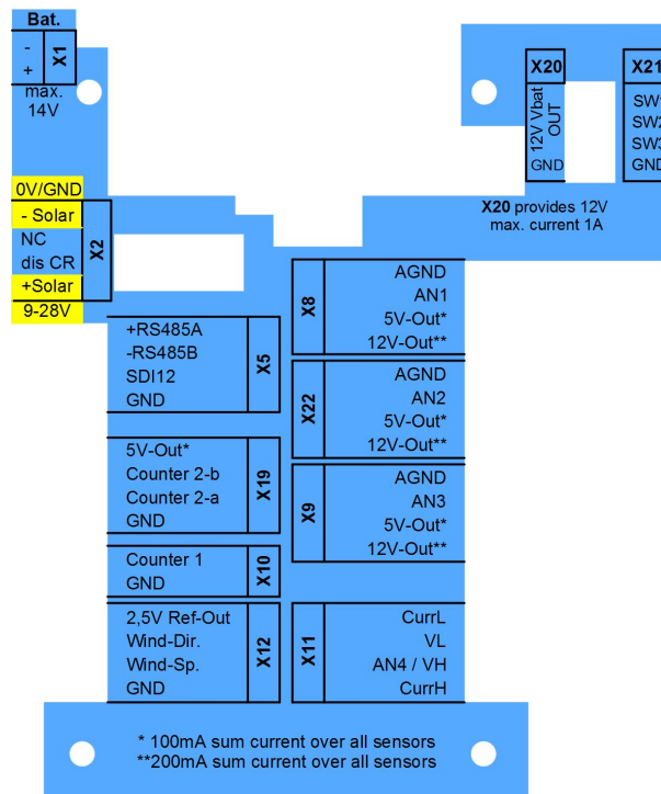
Abbildung 2 Anschlussklemmen des MRL-8P
