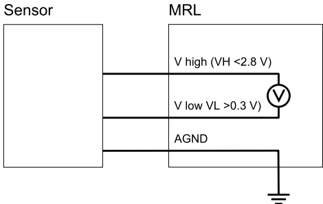
Abbildung 8 Interne Verdrahtung der analogen MRL-8E Eingänge
