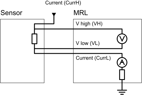
Abbildung 8 Interne Verdrahtung der analogen MRL-8E Eingänge
