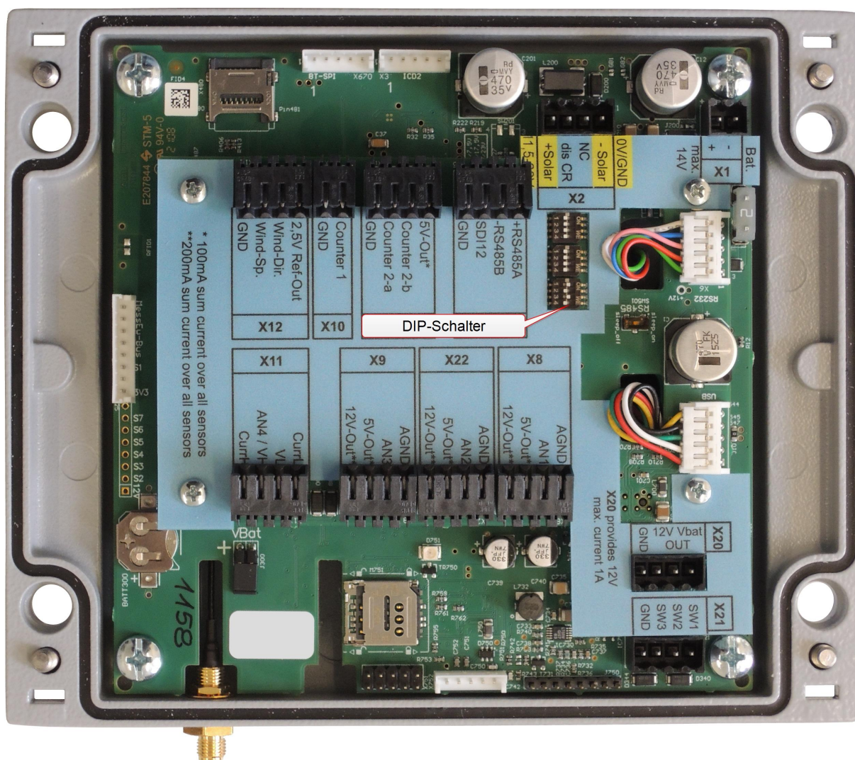
Abbildung 2 DIP-Schalter
