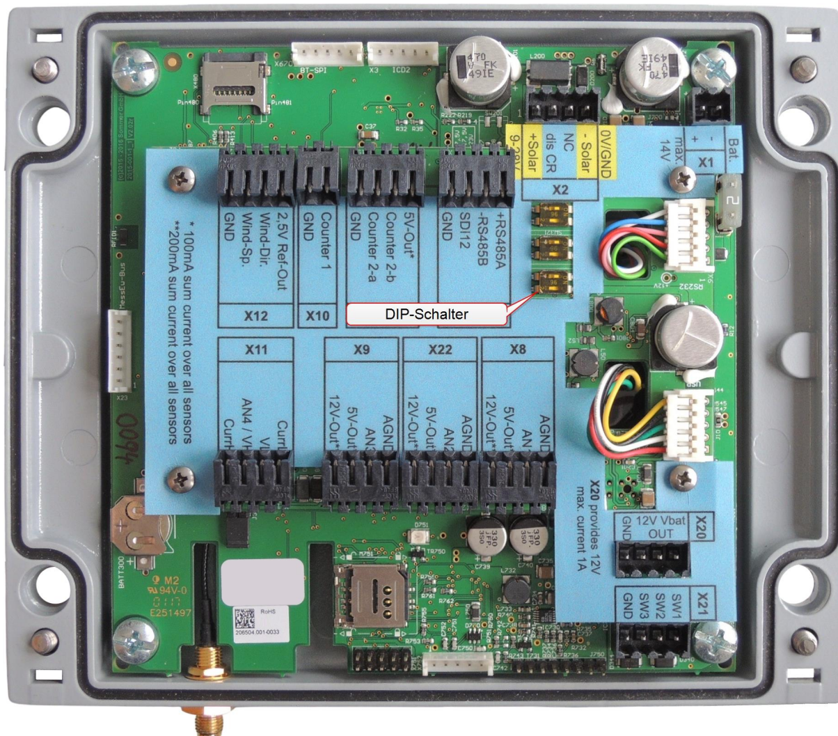
Abbildung 3 DIP-Schalter
