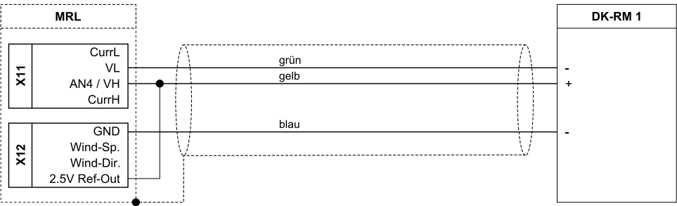
Abbildung 11 Verdrahtung einer differenziellen Spannungsmessung (Pyranometer)
