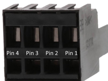
Abbildung 5 4-poliger Federclip
