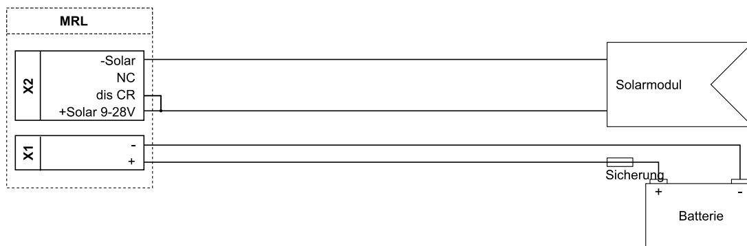
Abbildung 3 Verkabelung eines Solarmoduls
