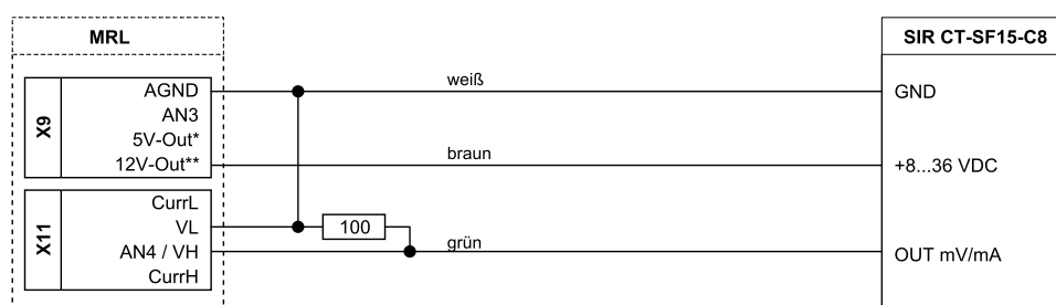
Abbildung 12 Verdrahtung eines Sensors mit Stromausgang (Infrarot-Temperatursensor)
