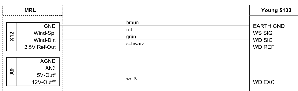
Abbildung 15 Verkabelung eines Frequenzeingangs (kombinierter Windgeschwindigkeits-/richtungssensor)
