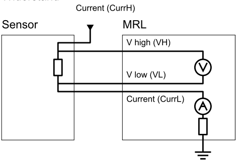
Abbildung 8 Interne Verdrahtung der analogen MRL-8B Eingänge
