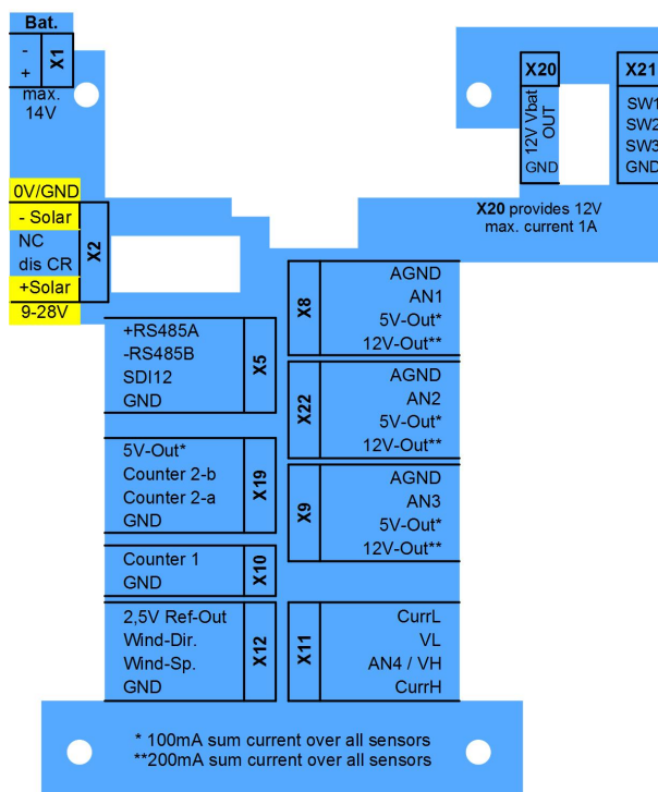
Abbildung 2 Anschlussklemmen des MRL-8B
