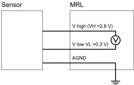
Abbildung 8 Interne Verdrahtung der analogen MRL-8B Eingänge
