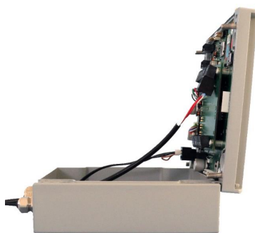
Abbildung 4 Öffnen Sie das MRL-8B-Gehäuse
