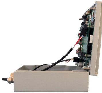
Abbildung 4 Öffnen Sie das MRL-8-Gehäuse
