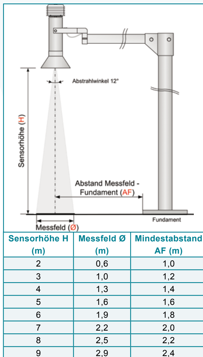
Abb. 2: Übersicht der Montagemaße des USH-8 Sensors.
