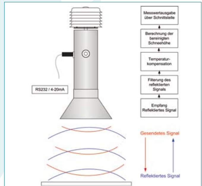
Abb. 1: Signalverarbeitung des USH-8 Schneehöhensensors.
